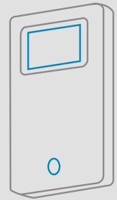
Käyttäjän pääte
